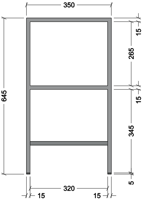
PROSPETTO FRONTALE
