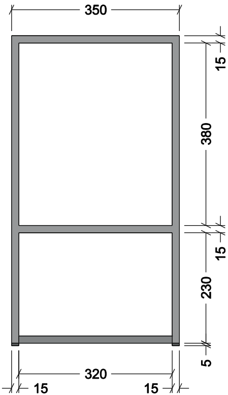
PROSPETTO LATERALE
