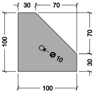
PIASTRA SALDATA SPESSORE 3 mm.
