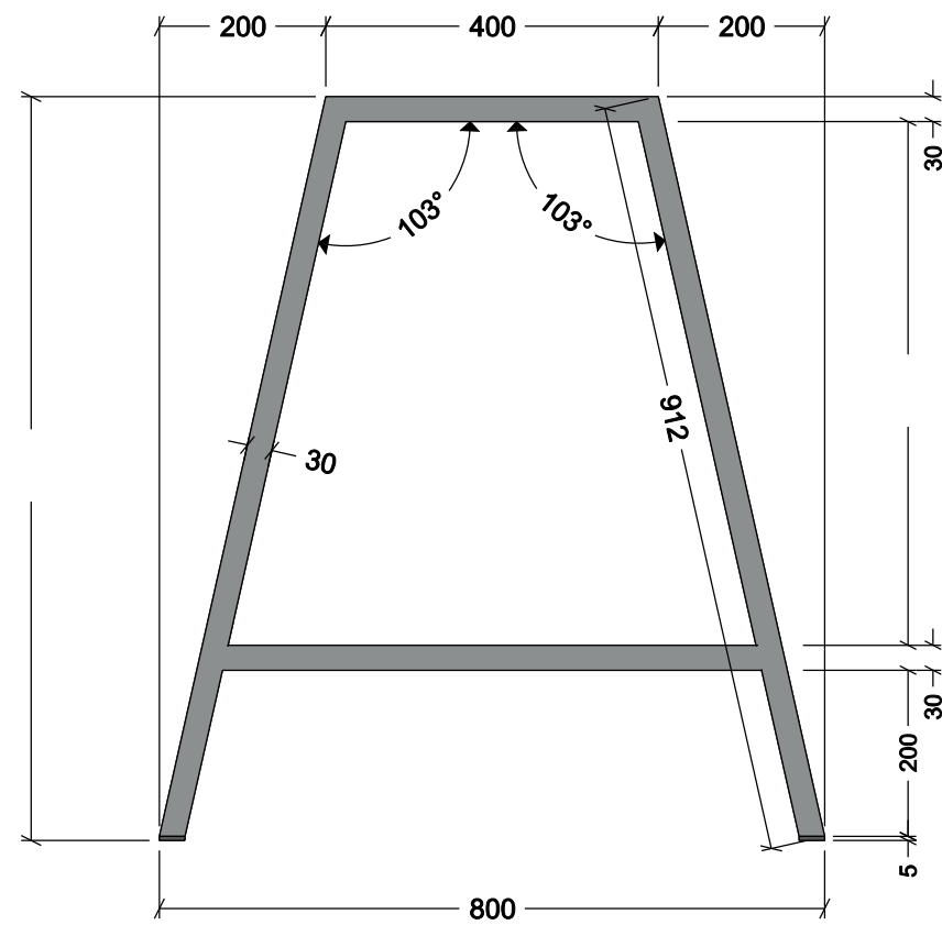
PROSPETTO FRONTALE
