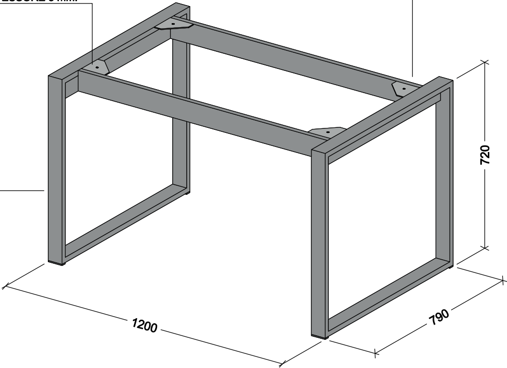
PIASTRA SALDATA SPESSORE 3 mm.
