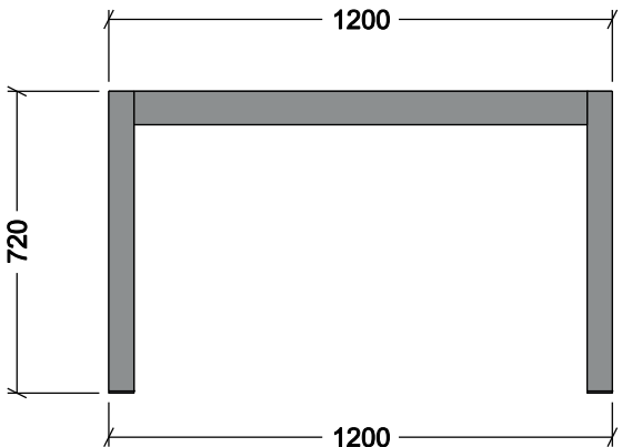
PROSPETTO FRONTALE
