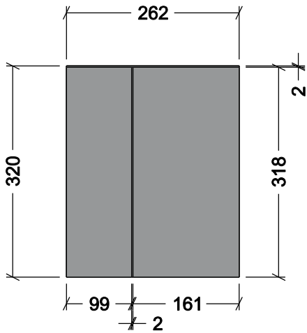
PROSPETTO FRONTALE
